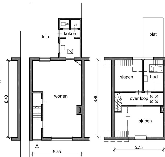
1:200 begane grond en eerste verdieping
